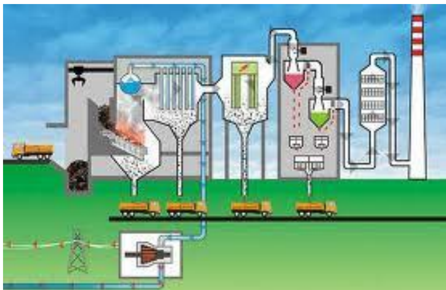
39. ábra Hulladéktüzelésű erőmű vázlata
